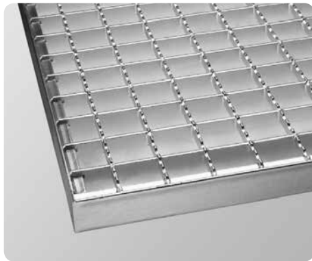
Typ PR/S3, zoubkovaný rozpěrný příčný pás
